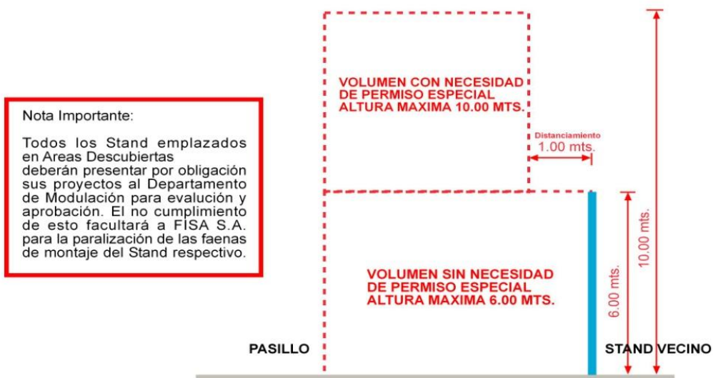
Esquema de elevación lateral
