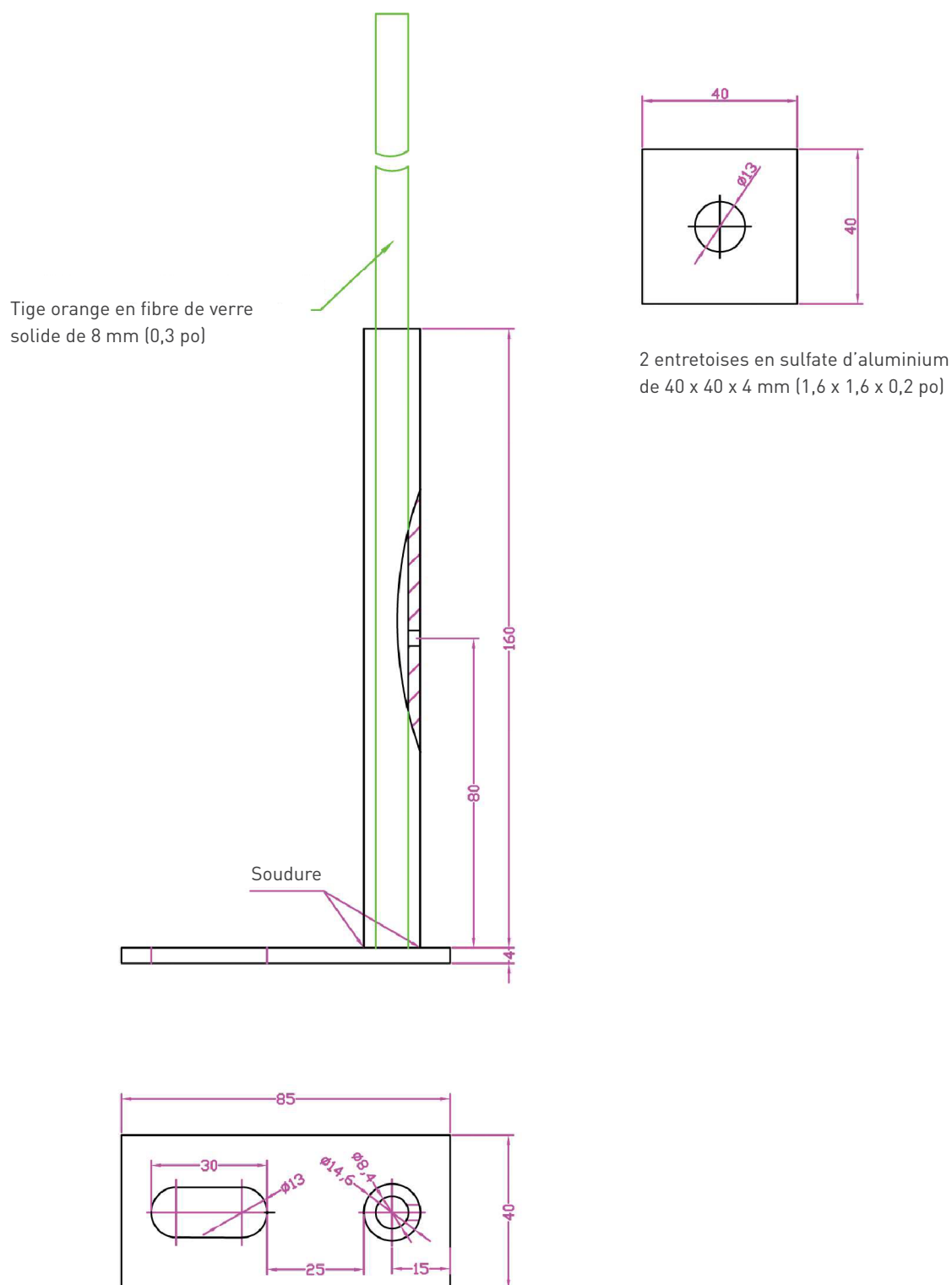
Fig. 1. Indicateur de dôme de drain
