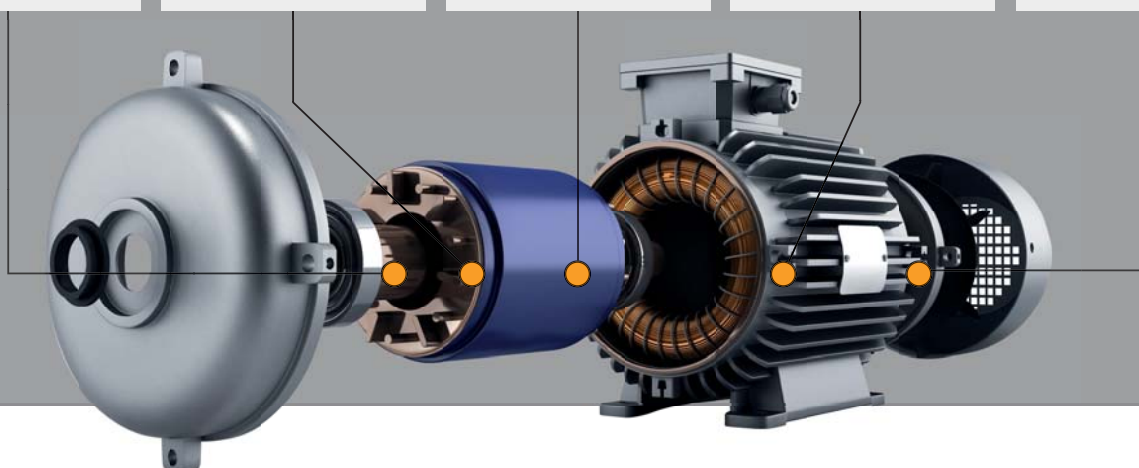
ROTOR: FÜGEN DER WELLE
