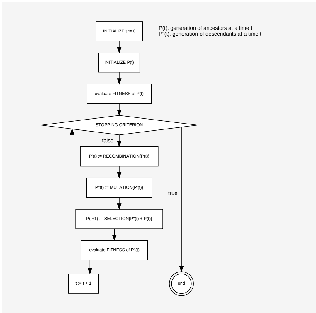
Figure 59.1. Structure d'un algorithme génétique
