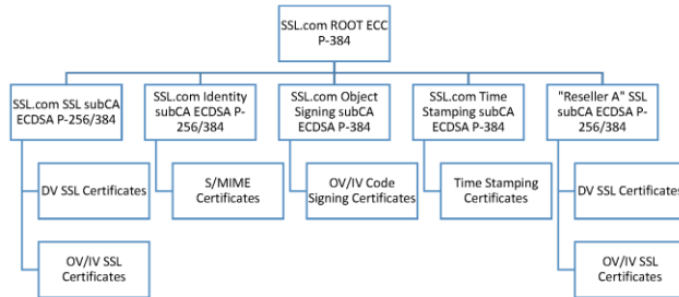
SSL.com ECC CA Hierarchy
