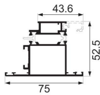
JNW-HC847A 75 new clip glass fan Weight : 1.39 kg/m
