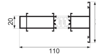
JNW-ZH762A center column Weight : 1.78 kg/m
