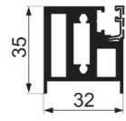
JNW-XT1464 mesh door bottom frame Weight : 1.30 kg/m
