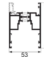
JNW-TS911F 75 lifting door Weight : 1.79 kg/m
