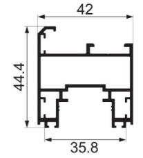
JY-42ZD-01 door frame Weight : 0.882 kg/m
