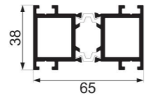
JY-75ZD-22 center column Weight : 0.865 kg/m
