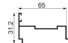
JY-75ZD-04 door frame closing Weight : 0.441 kg/m
