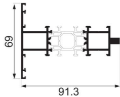
JNW-CT1251D center column Weight : 1.87 kg/m
