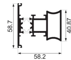
JY-58DQ-01 + JY58DQ-02 big center column Weight : 0.584 kg/m , 1.183 kg/m
