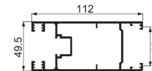
JNW-A-006 112 vertical door frame Weight : 2.27 kg/m
