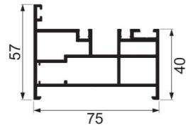
JY-75ZD-02 side frame Weight : 1.971 kg/m
