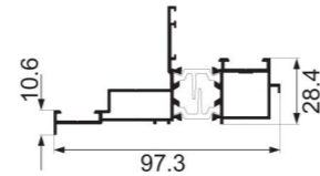
JNW-FK773A subframe Weight : 1.29 kg/m
