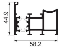
JY-58DQ-08 + JY-58DQ-07 small center column Weight : 0.478 kg/m , 1.117 kg/m
