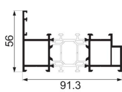
JNW-CT1249D outer frame Weight : 1.84 kg/m
