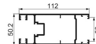
JNW-A-005 112 vertical door frame Weight : 1.92 kg/m
