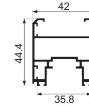
JY-42ZD-01 door frame Weight : 0.897 kg/m
