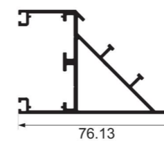
JY-50ZD-09 corner Weight : 1.23 kg/m
