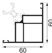
JNW-XT1009 90° slim corner Weight : 1.14 kg/m
