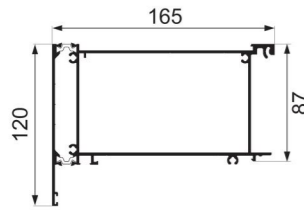
JNW-SJC22A 150 upper frame Weight : 4.04 kg/m
