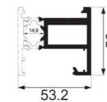
JNW-SJC039 glass door panel Weight : 2.05 kg/m
