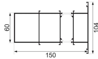
JNW-ZT802 strengthen inner frame Weight : 3.26 kg/m
