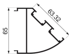
JY-75ZD-09 corner Weight : 1.081 kg/m
