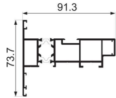
JNW-CT1728F flat sliding door Weight : 1.9 kg/m
