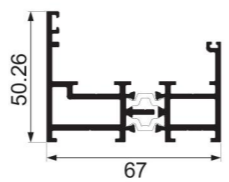
JY-58DQ-22 + JY-58DQ-21 side frame Weight : 0.959 kg/m , 0.689 kg/m
