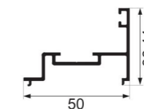
JY-50ZD-08 door frame closing Weight : 0.497 kg/m
