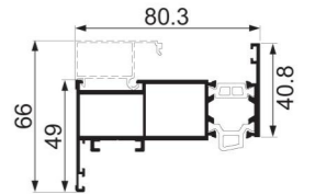
JNW-HC807A double inside out glass fan Weight : 1.65 kg/m
