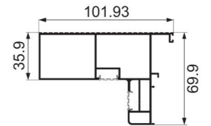
JNW-XT1470 handrail Weight : 1.51 kg/m
