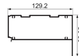
JNW-XT1185 intelligent top rail Weight : 2.16 kg/m
