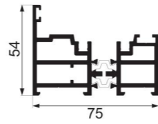
JY75ZD-38 + JY75ZD-37 side frame Weight : 1.140 kg/m , 0.914 kg/m
