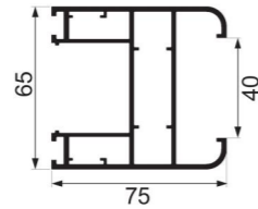
JY-75ZD-01 door frame Weight : 1.935 kg/m
