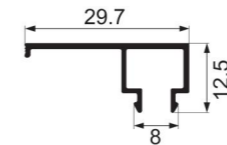
YC-SZ-5003 burclose 2 Weight : 0.152 kg/m
