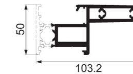
JNW-SJC31 strengthen glass door Weight : 3.25 kg/m
