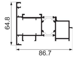
JNW-CT1725F flat sliding sub-frame Weight : 1.74 kg/m
