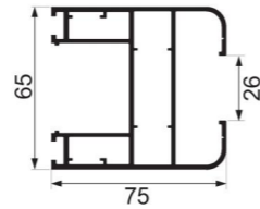
JY-75ZD-07 door frame Weight : 1.923 kg/m
