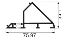
JY-58DQ-17 + JY-58DQ-18 corner Weight : 0.198 kg/m , 0.910 kg/m
