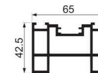
JY-75ZD-27 door frame Weight : 1.890 kg/m
