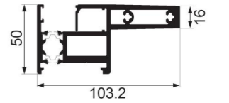
JNW-SJC23 strengthen glass door Weight : 3.39 kg/m
