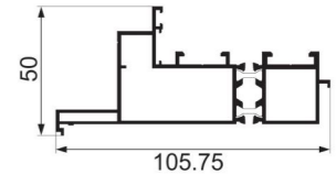
DZ-CT797F slim subframe Weight : 1.55 kg/m
