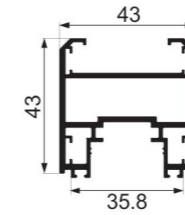
JY-42ZD-18 door frame Weight : 0.897 kg/m
