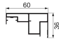
JNW-A-042 60 packs Weight : 0.77 kg/m
