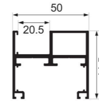
JY-50ZD-07 door frame Weight : 1.1 kg/m
