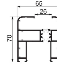
JY-75DQ-01 + JY-75DQ-02 sash frame Weight : 1.201 kg/m , 0.918 kg/m
