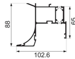
JNW-SJC24A screen upper frame Weight : 2.29 kg/m
