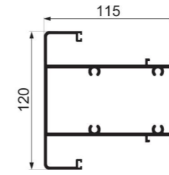
JY-120-13 door frame center cross Weight : 4.244 kg/m
