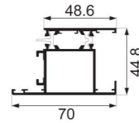
JNW-HC771A 3 glass fan Weight : 1.31 kg/m
