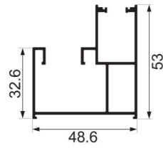
JY-50TS-01A side frame Weight : 0.798 kg/m
