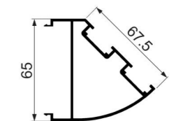
JY-75ZD-09 corner Weight : 1.081 kg/m
