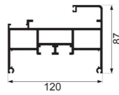
JY-120-05 door frame Weight : 4.303 kg/m
