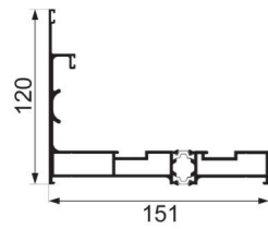
JNW-SJC26A 150 side frame Weight : 3.34 kg/m
