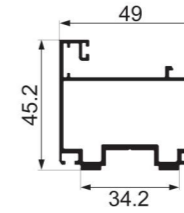
YC-SZ-6002 60 door frame Weight : 0.873 kg/m
