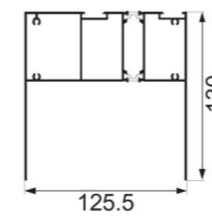
JNW-CT1584F 128 intelligent top rail Weight : 2.95 kg/m
