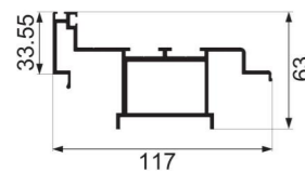
JY-120-09 door frame closing Weight : 2.017 kg/m
