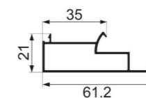
JY-42ZD-16 clip Weight : 0.469 kg/m
