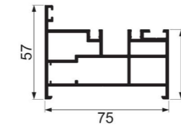
JY-75ZD-17 side frame Weight : 1.918 kg/m
