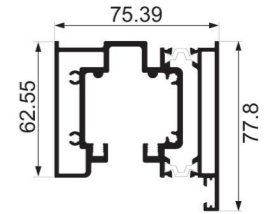
JY-75DQ-05 + JY-75DQ-06 hanging rail Weight : 2.224 kg/m , 0.900 kg/m
