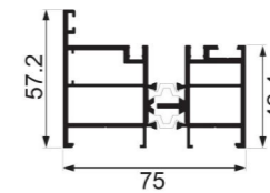
JY-75DQ-03 + JY-75DQ-04 out frame Weight : 1.117 kg/m , 0.958 kg/m
