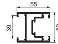
JNW-A-035 55 vertical door frame Weight : 1.82 kg/m
