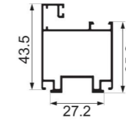
YC-SZ-4502 45 door frame Weight : 0.596 kg/m
