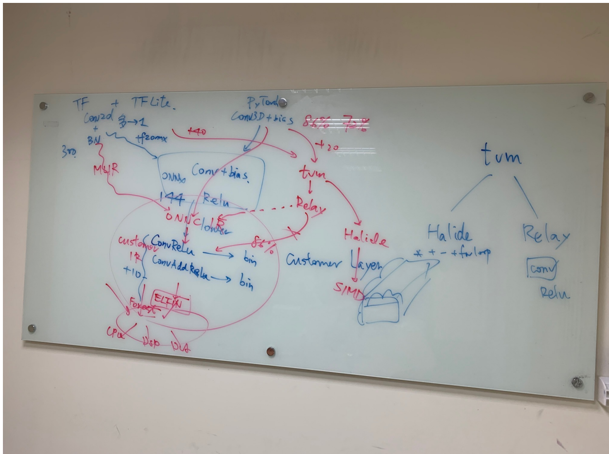
Fig. 16.1: ONNC
