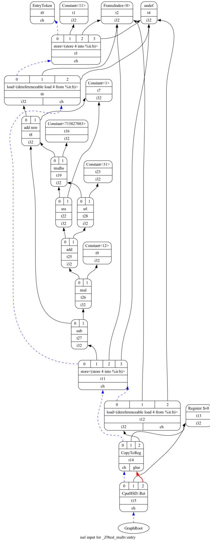
Fig. 4.2: ch4_1_mult.bc DAG
