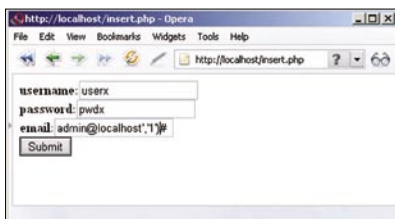
Abbildung 7. Benutzer mit Administratorstatus erstellen.
