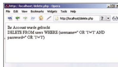
Abbildung 9. Alle Benutzer löschen
