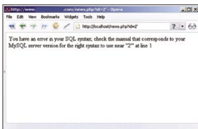
Abbildung 1. Fehlererzeugung durch Einfügen von einfachen Anführungszeichen
