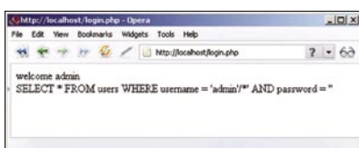
Abbildung 4. Bypass Login durch SQL Injection 2
