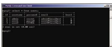
Abbildung 2. Auflistung von Benutzern in der users Tabelle
