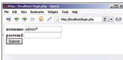
Abbildung 3. Bypass Login durch SQL Injection
