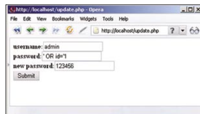
Abbildung 8. Passwort aktualisieren ohne das alte Passwort zu kennen
