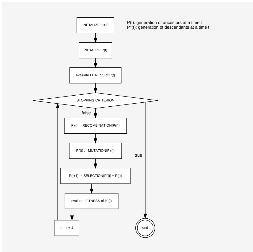
Figure 62.1. Structure d'un algorithme génétique
