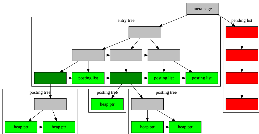
Figure 70.1. Cœur de GIN
