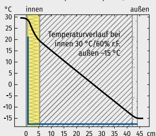
Grafik 1 normal, U-Wert 0,24 W/m²K
