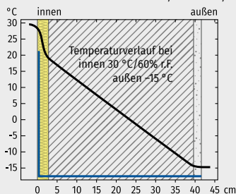
Grafik 2 Passivhaus-Standard, U-Wert 0,15 W/m²K
