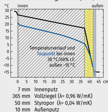
Grafik 3 vor Sanierung, U-Wert 0,55 \text{ W/m}^2\text{K}
