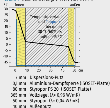
Grafik 4 nach Sanierung, U-Wert 0,24 \text{ W/m}^2\text{K}
